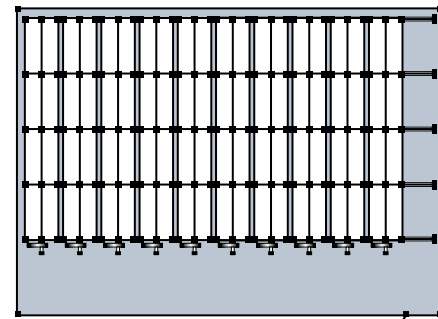
Увеличение вместимости архива вдвое при сохранении площади. Мобильный архив, площадь 40 кв. метров, 4200 единиц хранения. Единица хранения – папка типа «Корона» шириной 70 мм.
